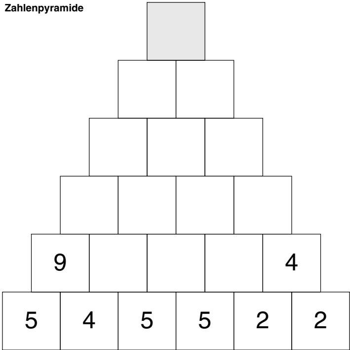
Zahlenpyramide
